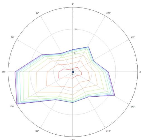
Róża wiatrów sezon roczny Stacja meteorologiczna: Toruń
